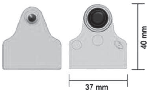
Rozměry M malá známka
