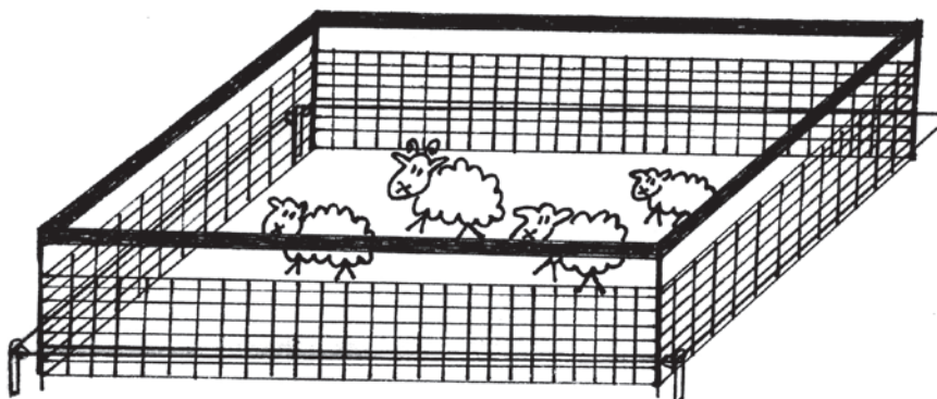
Obr. 3. pevný drátěný ohradník (výška min. 120 cm, lépe 140 cm), páska 20-30 cm nad ohradníkem opticky brání přeskočení ohrady, elektrický drát (min. 2 500 V) okolo ohrady cca 20 cm nad zemí brání podhrabání (proti podhrabání se dá také zapustit pevný drátěný ohradník min. 50 cm pod zem, nebo použít drátěné pletivo navazující na ohradník v úrovni země o šířce min. 100 cm)
