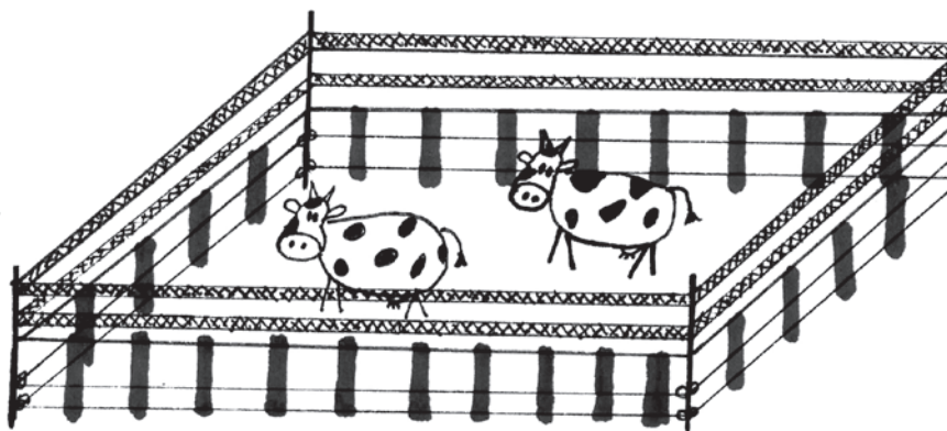
Obr. 4. zradidlový ohradník , zradidla jsou pruhy červené látky na laně umístěné max. 50 cm od sebe, dosahují k zemi nebo max. 20 cm nad zem, dva elektrické dráty dole cca 20 cm nad zemí brání podhrabání/podlezení, pásky 20-30 cm nad zradidlovým ohradníkem opticky brání přeskočení ohrady (jednoduchý fladrový ohradník bez přídatných opatření slouží jen dočasně, cca 1-2 měsíce, poté si vlci zvyknou)
